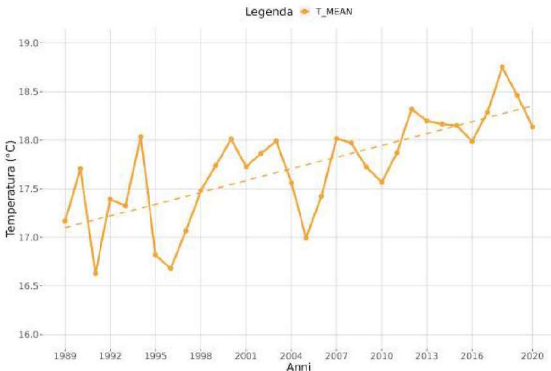
Figura 5.11: Indice climatico TMEAN | temperatura media annua (C°). Fonte CMCC (Centro Mediterraneo Cambiamento Climatico)
