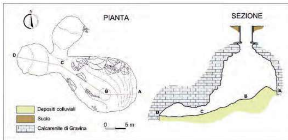
Figura 5.19: Pianta e sezione di una Vora (da AA.VV. 2008)
