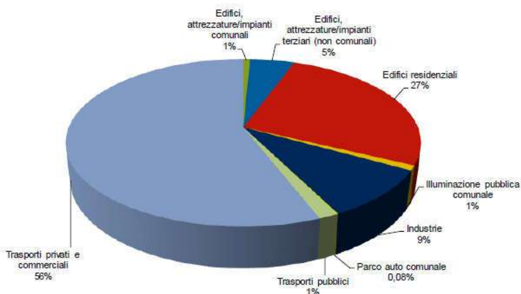
Figura 3.3: Ripartizione dei consumi energetici totali per categoria
