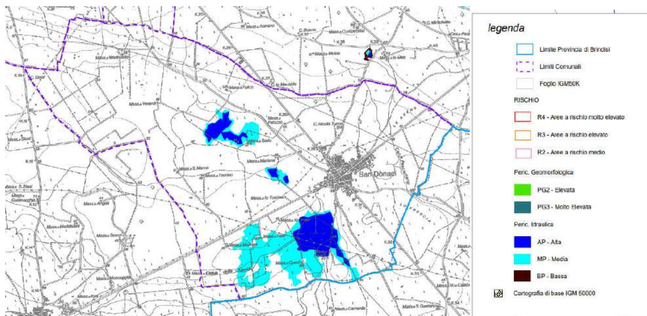
Figura 5.29: PAI Regione Puglia - Perimetrazione delle aree a pericolosit  idraulica e a rischio idraulico
