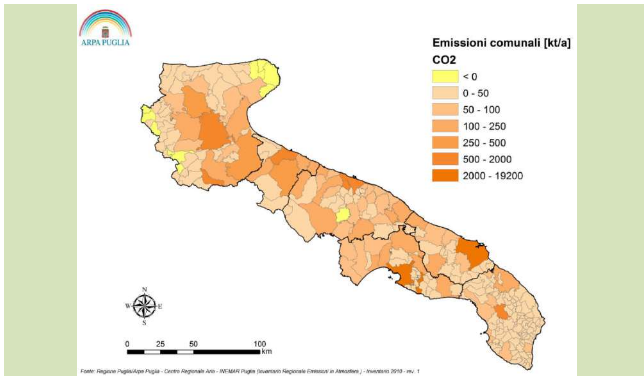
Figura 3.2: Emissioni comunali di CO 2 della Regione Puglia
